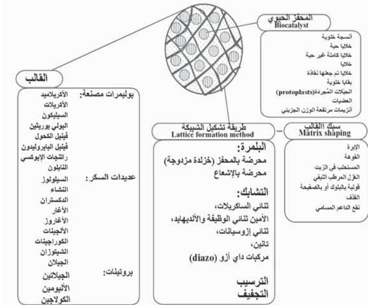
الشكل 5.24: لمحة عامة عن احتجاز المحفزات الحيوية بالشبكة
